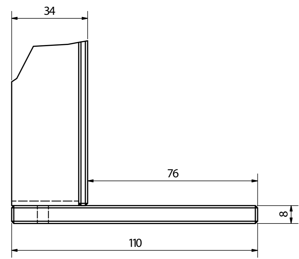
A ( 1 : 1 )
