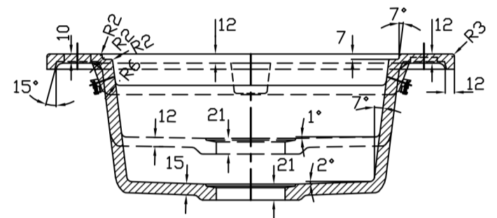
REZ B-B
