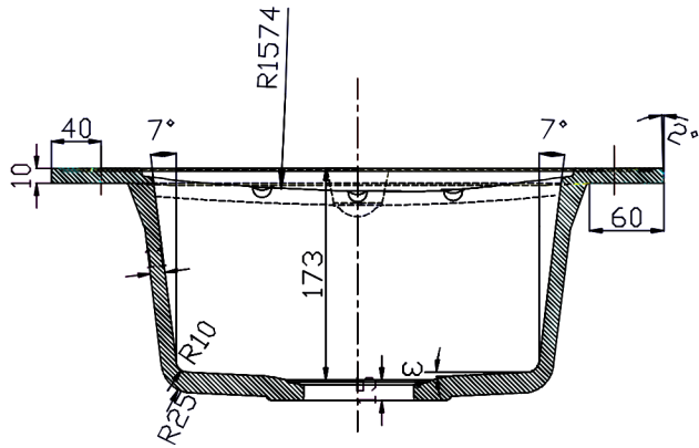
REZ B-B
