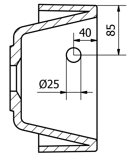
B-B ( 1 : 4 )
