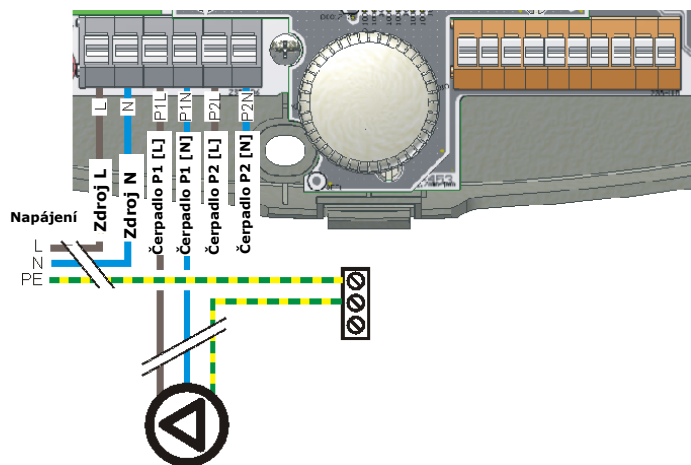
Obr. 17.6 Připojení čerpadel
