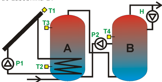
Obr. 14.4 Schéma zapojení D
