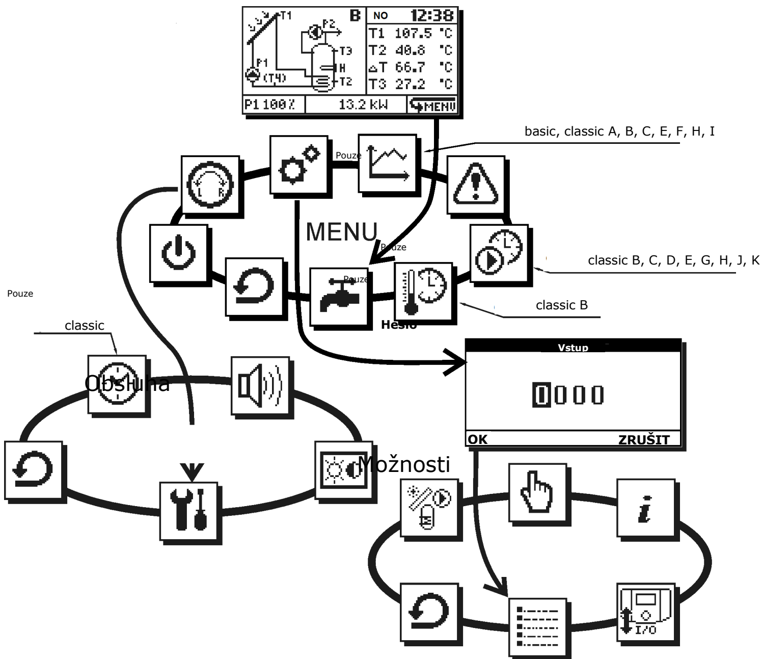
Obr. 7.5 Struktura menu regulátoru
