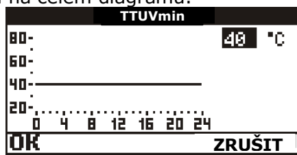
Obr. 9.1 Nastavení hodnoty TzTTUVmin
