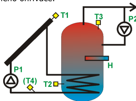
Obr. 14.2 Schéma zapojení B
