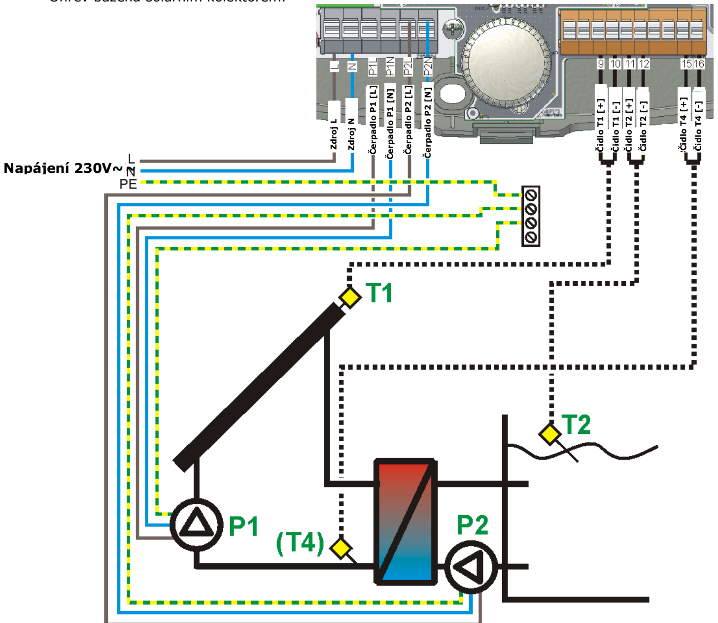
Obr. 18.8 Schéma zapojení I
