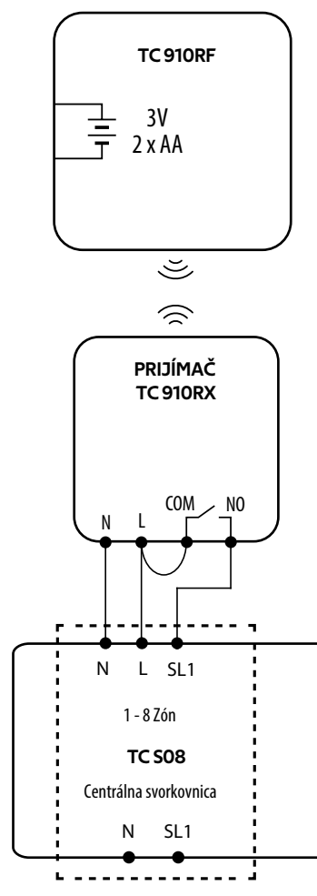
c) Schéma pripojenia k centrálnej svorkovnici
