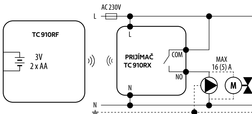
b) Schéma pripojenia k čerpadlu / pohonu
