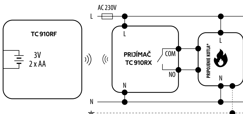
a) Schéma zapojenia plynového kotla
