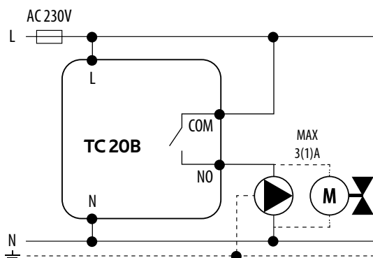
b) Schéma pripojenia k čerpadlu / pohonu
