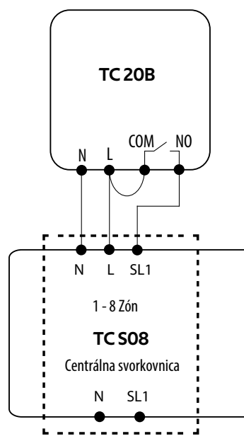
c) Schéma pripojenia k centrálnej svorkovnici
