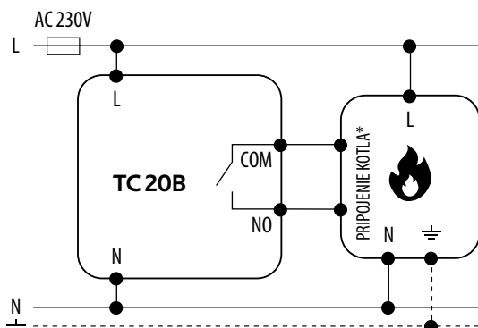
a) Schéma zapojenia plynového kotla
